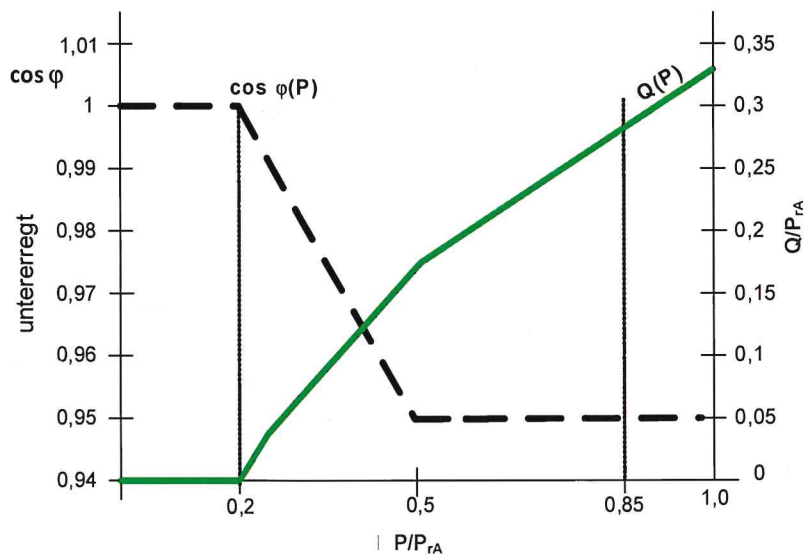
Bild 3 Q = f(P/P_{rA}) -Kennlinie für EZA mit P_{rA} \geq 135 \text{ kW} und Anschluss in den Umspannungsbereichen Königsbrück, Kamenz, Zescha, Kleinsaubernitz, Niesky, Görlitz und Weinhübel
