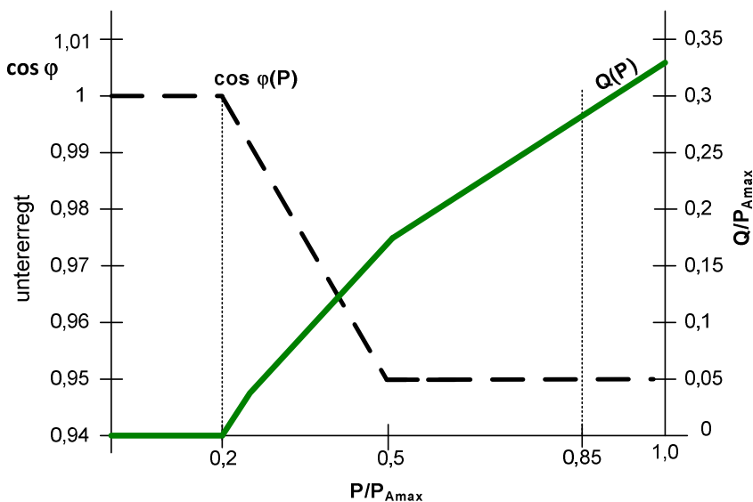
Bild 2 Q = f(P/P_{Amax}) -Kennlinie für Erzeugungsanlagen mit P_{Amax} \geq 135 \text{ kW} und Anschluss in den Umspannungsbereichen Königsbrück, Kamenz, Zescha, Kleinsaubernitz, Niesky, Görlitz und Weinhübel
